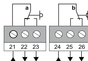
Interruttori ausiliari
